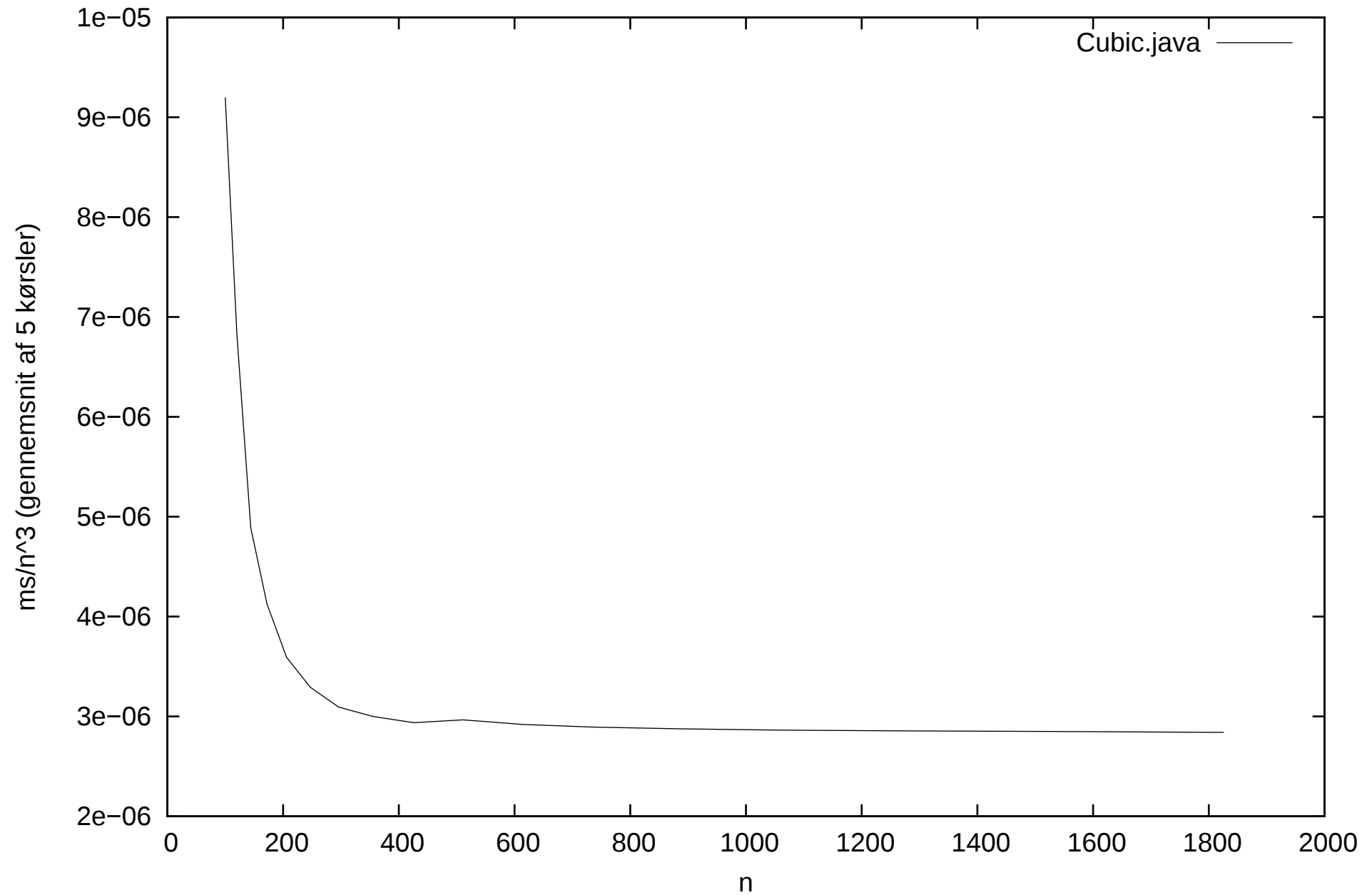
Cubic.java, plot af (\text{målt tid})/n^3
