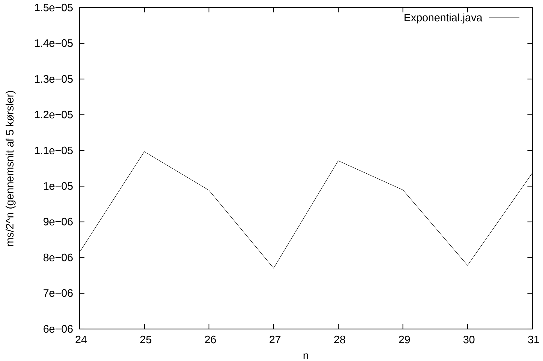
Exponential.java, plot af (målt tid)/2 n
