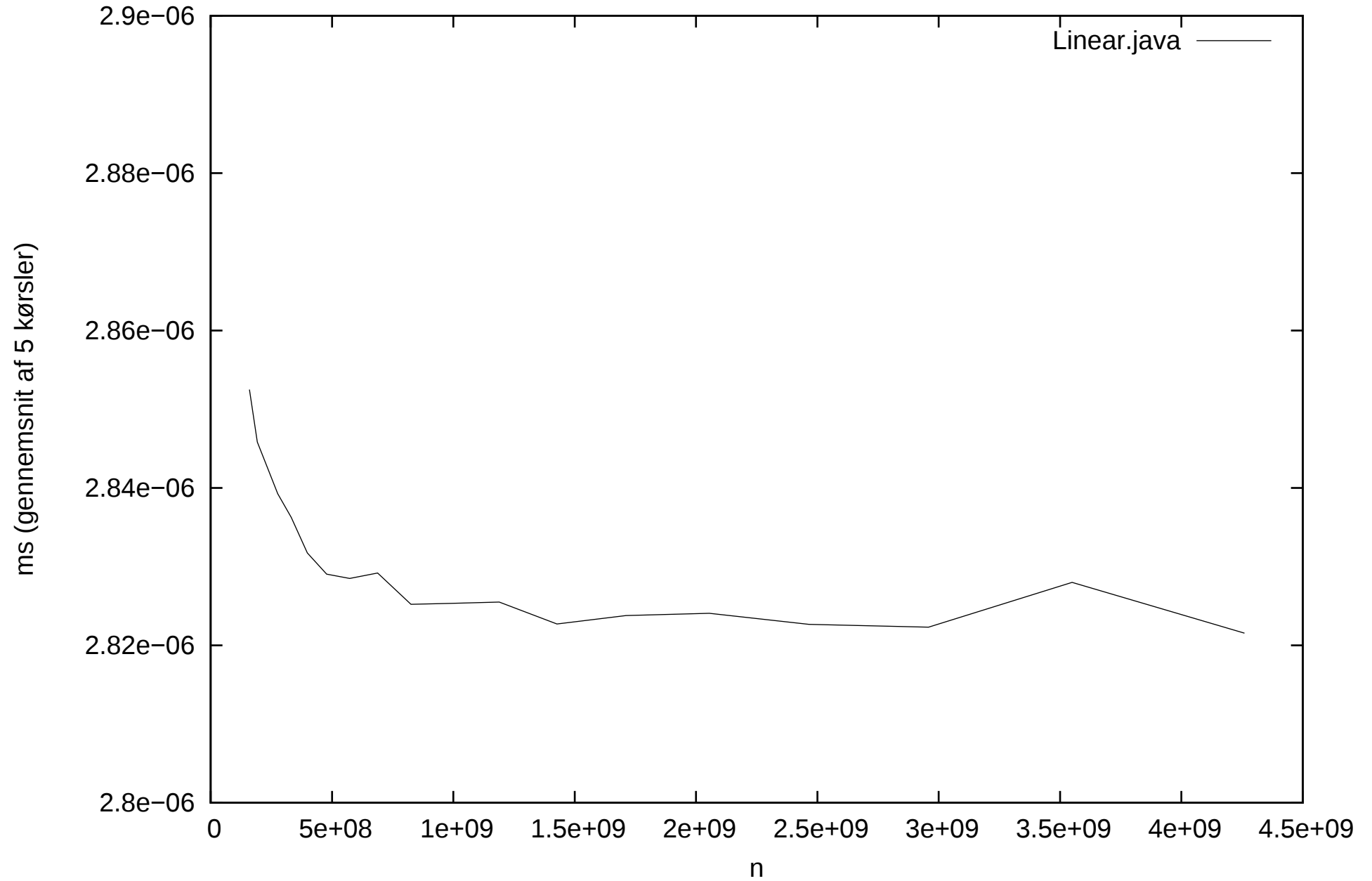
Linear.java, plot af (målt tid)/n
