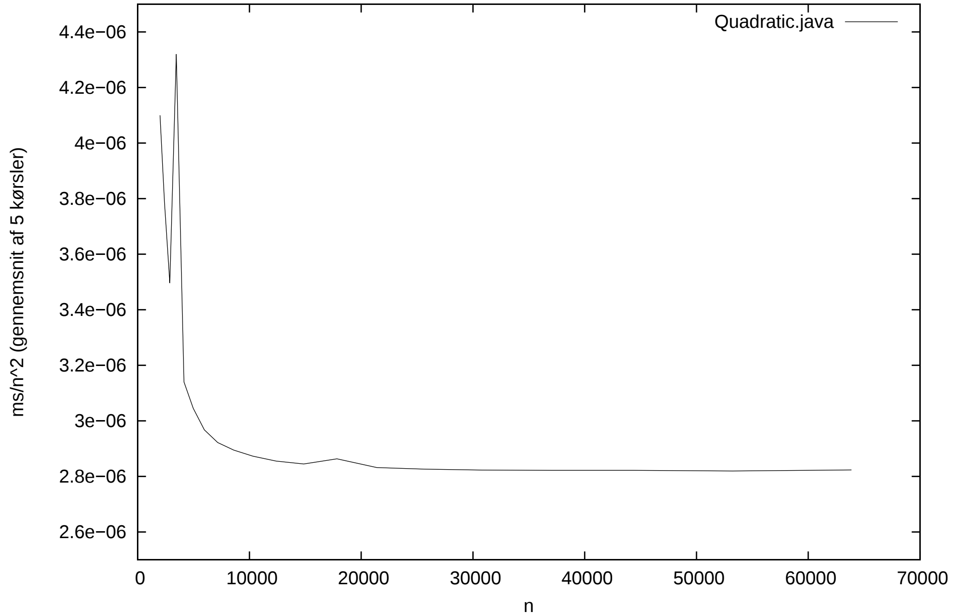
Quadratic.java, plot af (målt tid)/n^2
